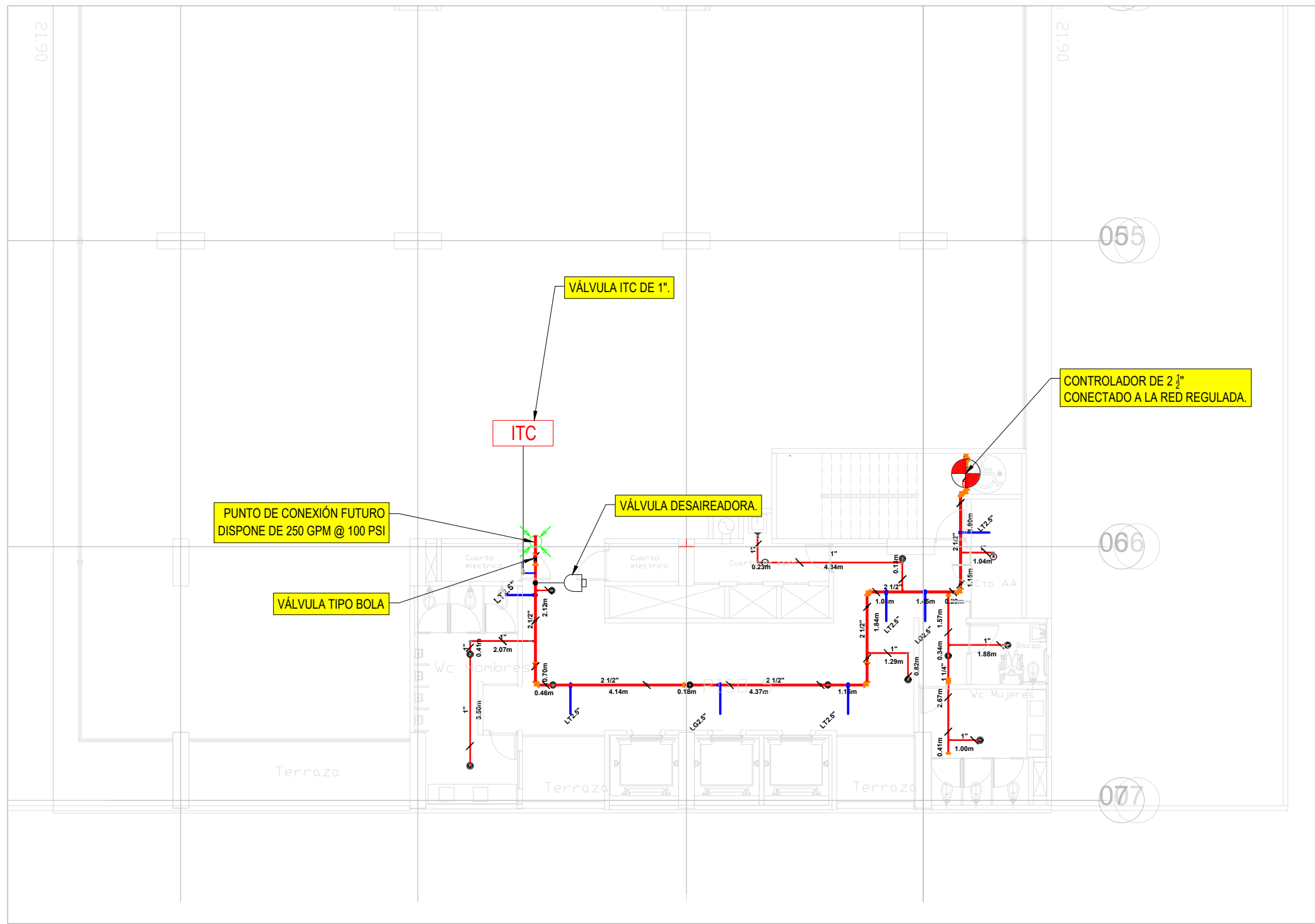
1 VISTA EN PLANTA EXTINCIÓN PISO 5 ESCALA 1:150
