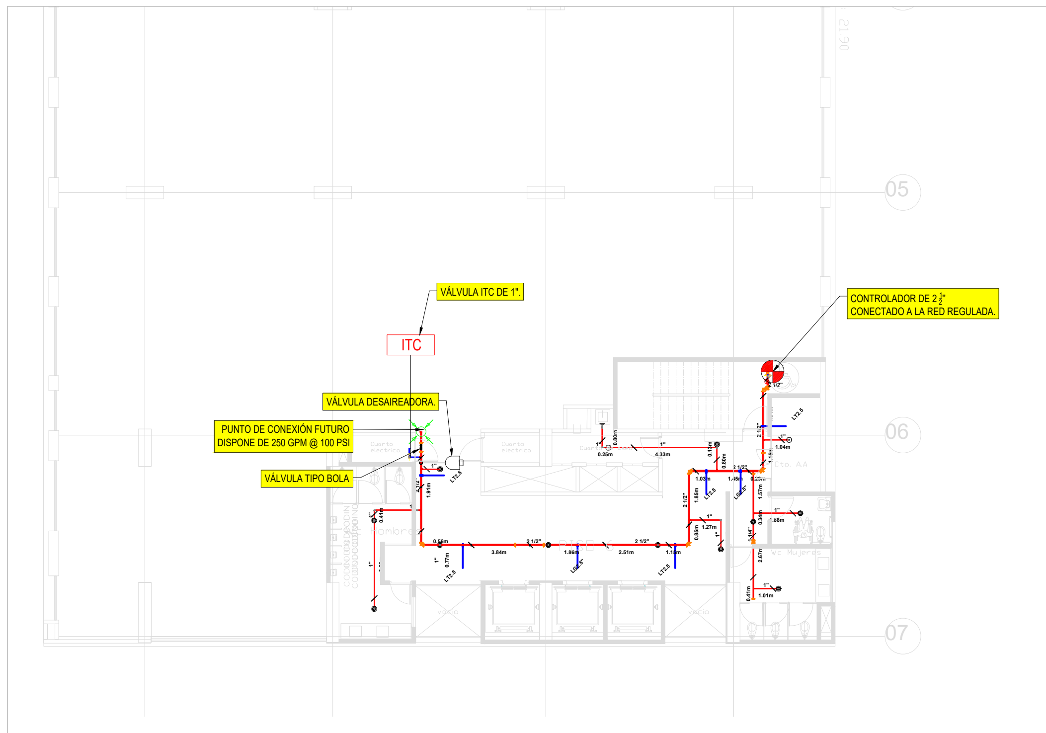
4 VISTA EN PLANTA EXTINCIÓN PISO 8 ESCALA 1:150
