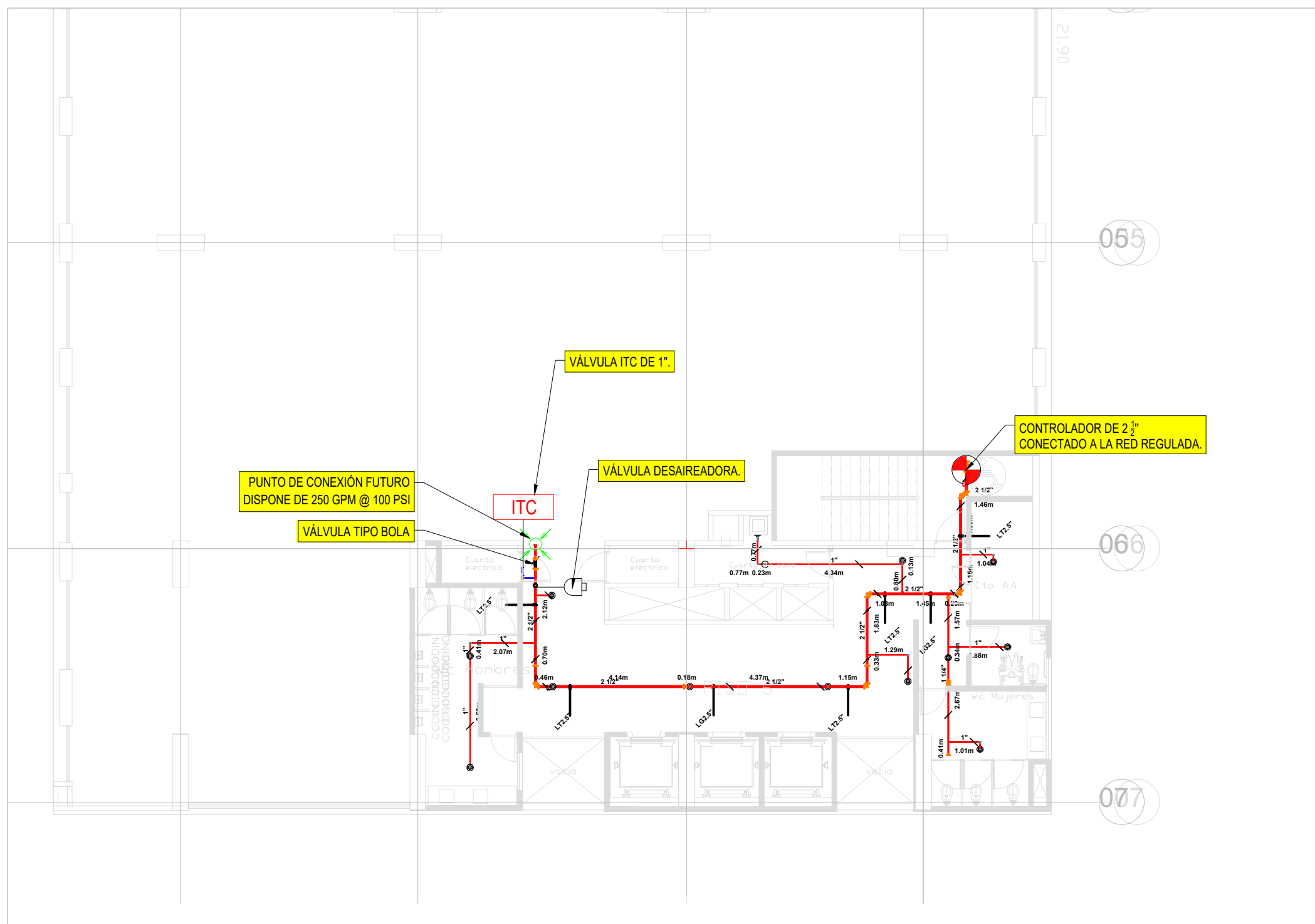
2 VISTA EN PLANTA EXTINCIÓN PISO 6 ESCALA 1:150
